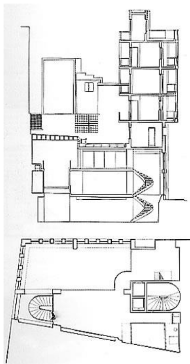
Εικ. 2.1, 2.2, 2.3.: Απόψεις του εκθεσιακού χώρου, της κάτοψης και της τομής από το Μουσείο Φασιανού. Πηγή: http://www.culture2000.tee.gr/ATHENS/GREEK/BUILDINGS/BUILD_TEXTS/B104_t.html και https://www.huffingtonpost.gr/entry/to-moeseio-alekoe-fasianoe-dinei-neo-pnoe-sto-kentro-tes-athenas_gr_6139f8e8e4b0640100a167fa (τελευταία επίσκεψη: 01/02/2022).
